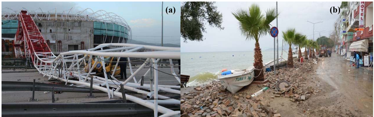
Şekil 2. (a) Bursa’da lodos’ta devrilen kule vincin görünümü [3] (b) Bursa’da Rüzgarda zarar gören sahil [4]
