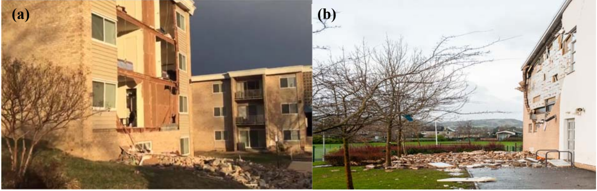
Şekil 4. (a) ABD’de şiddetli rüzgarda meydana gelen duvar hasarı [7] (b) İskoçya’da fırtına sonrası duvar hasarı [8]
