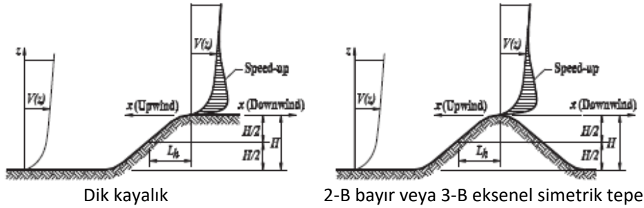
Şekil 8. Tepe ve bayırlarda rüzgar hızında meydana gelen artış (ASCE 7-10)
