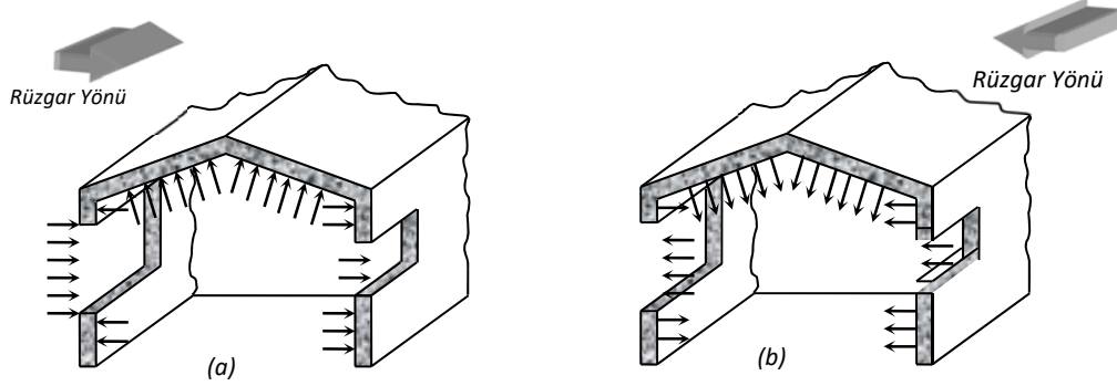
Şekil 7. Giriş/çıkış açıklık alanına göre rüzgar etkisinin değişimi
